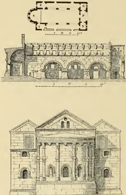
10580. — Plan, élévation, coupe et restauration de la basilique de Qalb-Louzé. D'après de Vogüé, Syrie centrale , Architecture, pl. CXXII-CXXVI.
